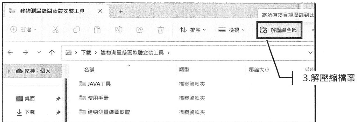
圖 4 解壓縮畫面
